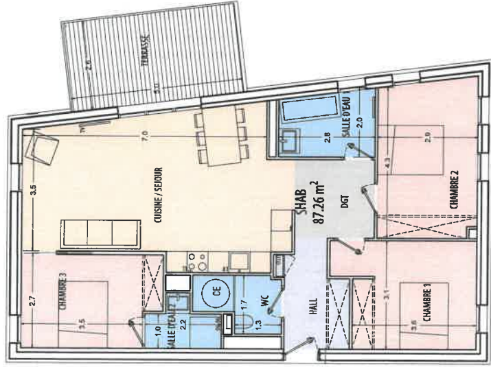
PLAN DE L'APPELLEMENT
