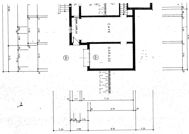
SOUS-SOL (éch: 1/100)
