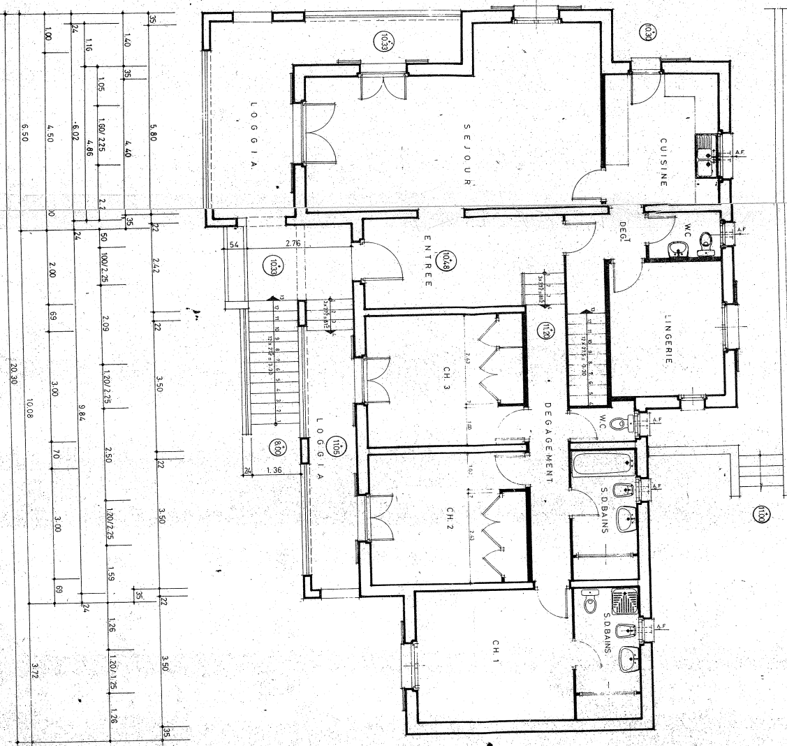
R.D.C.H. (éch: 1/50)
